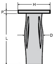
Nitonakrętka stalowa rozprężna M6
