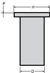
Nitonakrętka neoprenowa M5 x 26,5 z gwintem mosiężnym
