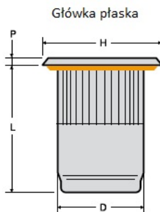
Nitonakrętka M10 szczelna zamknięta
